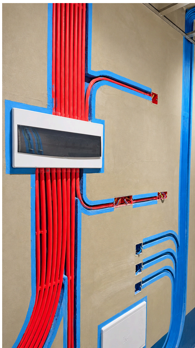
墙面电气线管施工
