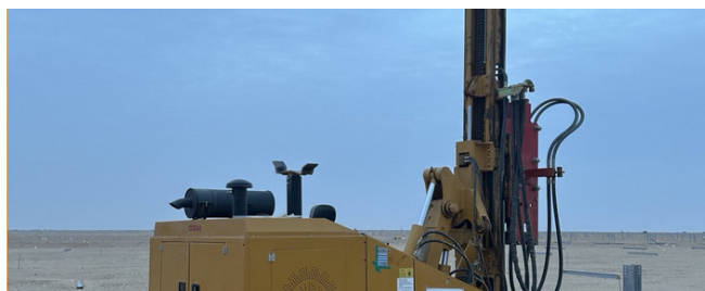
光伏桩基施工设备
